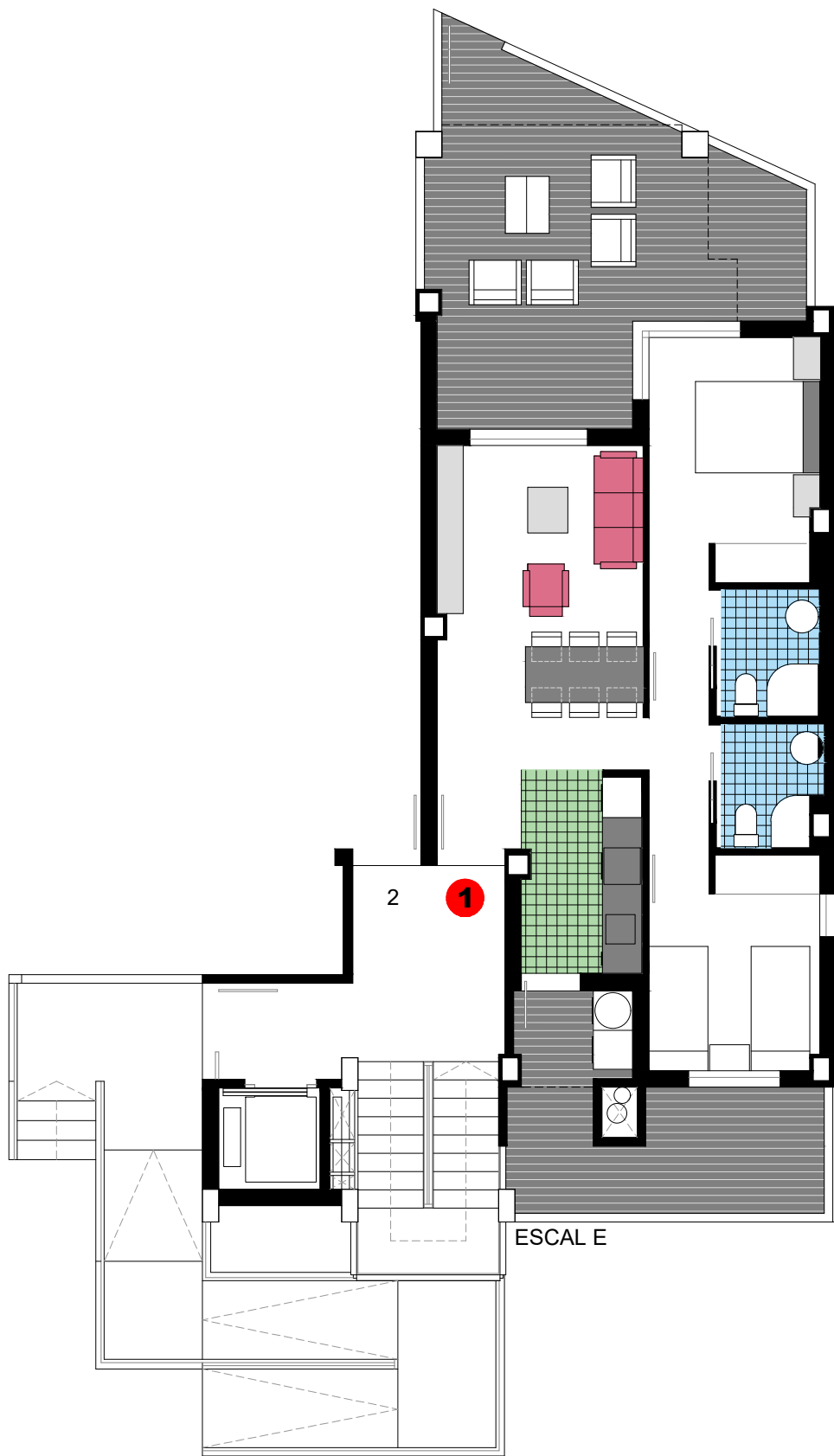
PLANTA BAJA
